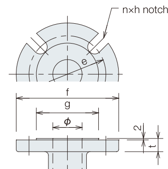
FLANGE
